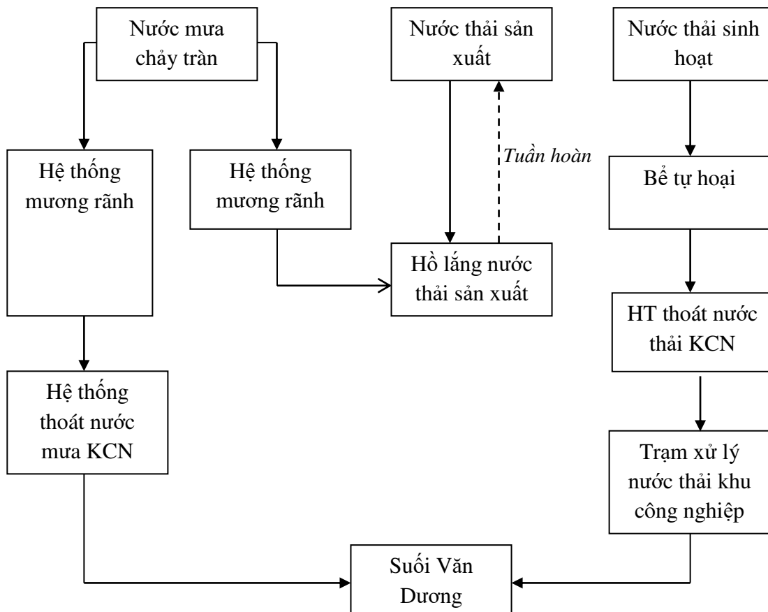
Hình 3. 1. Mạng lưới thu gom nước mưa, nước thải của nhà máy
